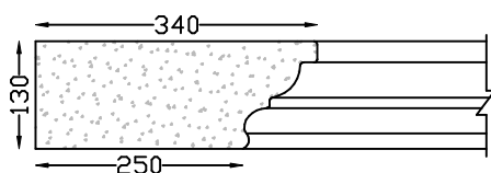
OG MINOR MK2 COPING Length 1,000m
